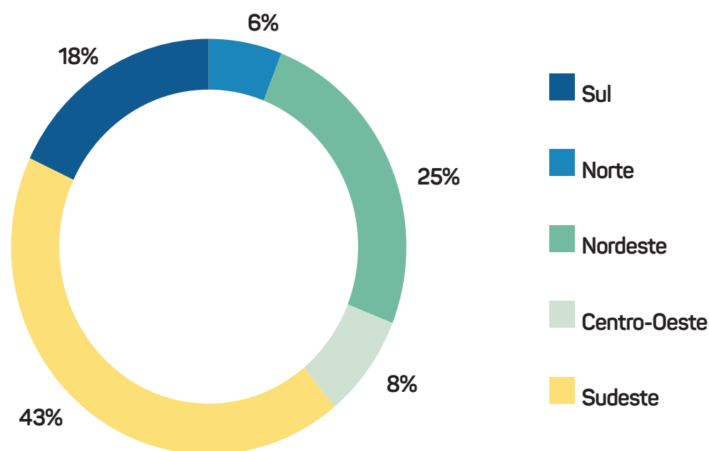
Gráfico 26. Percentual da geração de lodo de ETA por região.
